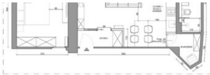
PLAN PROJET
