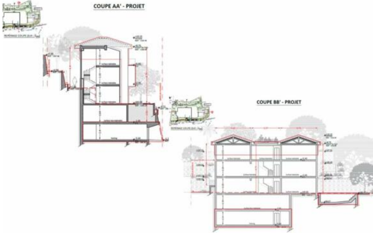
VILLA MY SOUL - VUE EN COUPE
