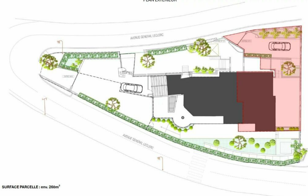
PLAN EXTERIEUR
