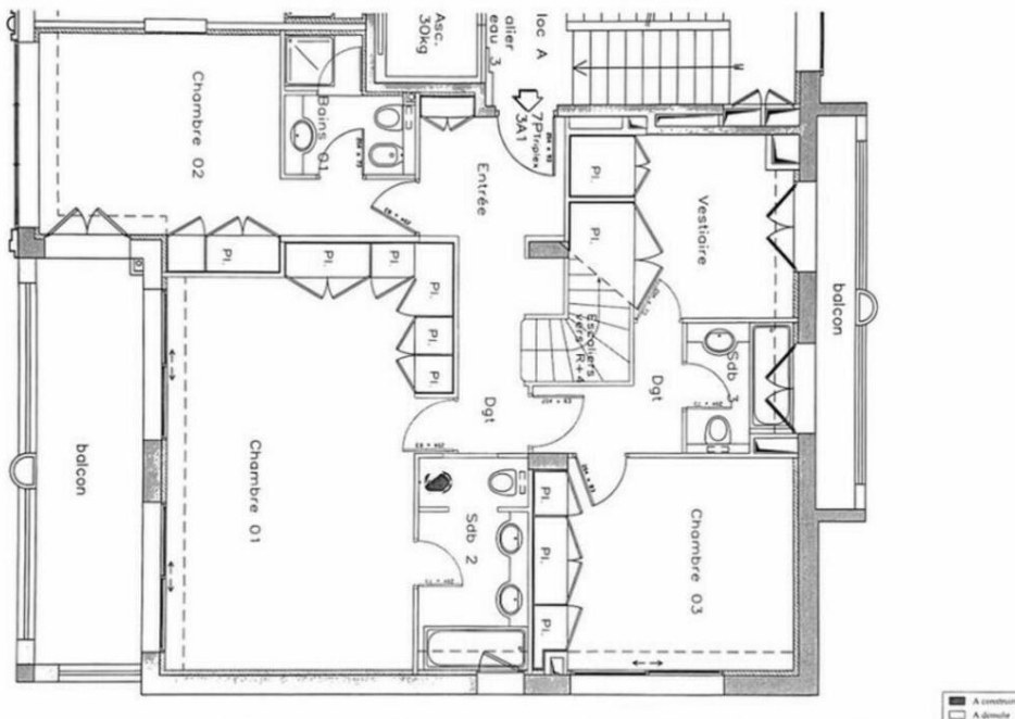
Plan modificatif - Appartements 3A1 + 4A1 - Niveau R+3
