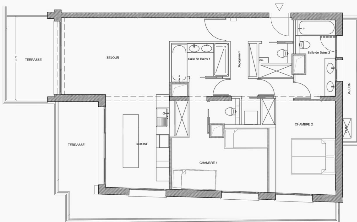
Plan Projet
